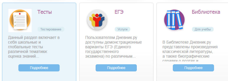
Рис.1. Управление разделами
